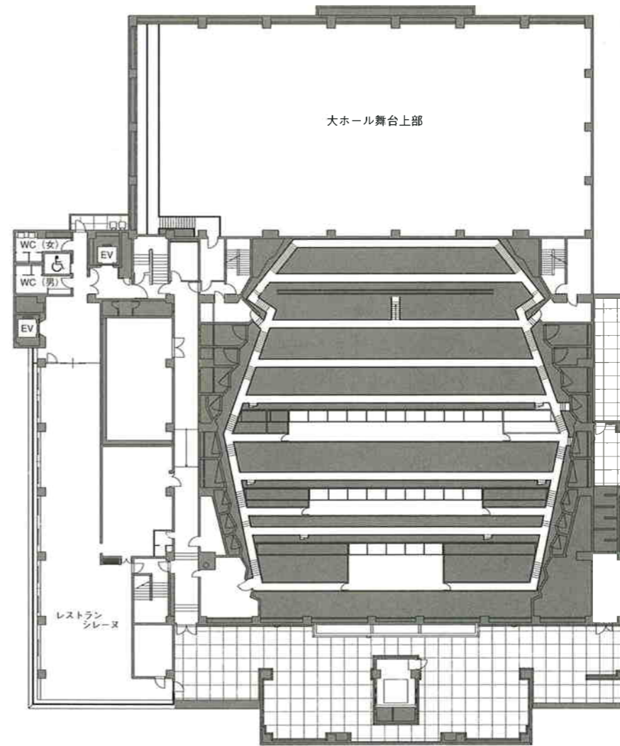
大ホール棟
