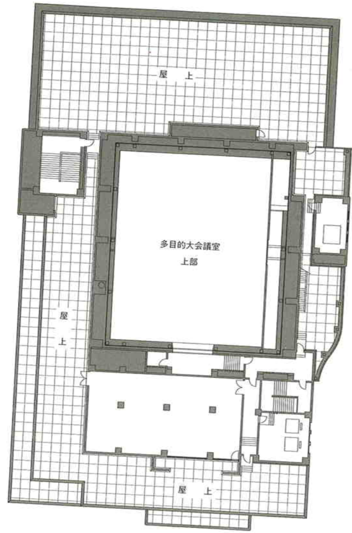
小ホール棟
